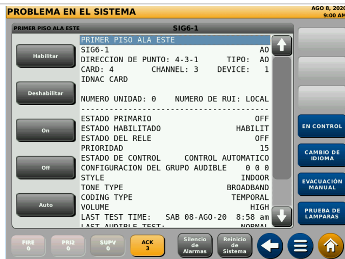
Figura 8: Pantalla de estado de punto detallado para dispositivo ES TrueAlert
