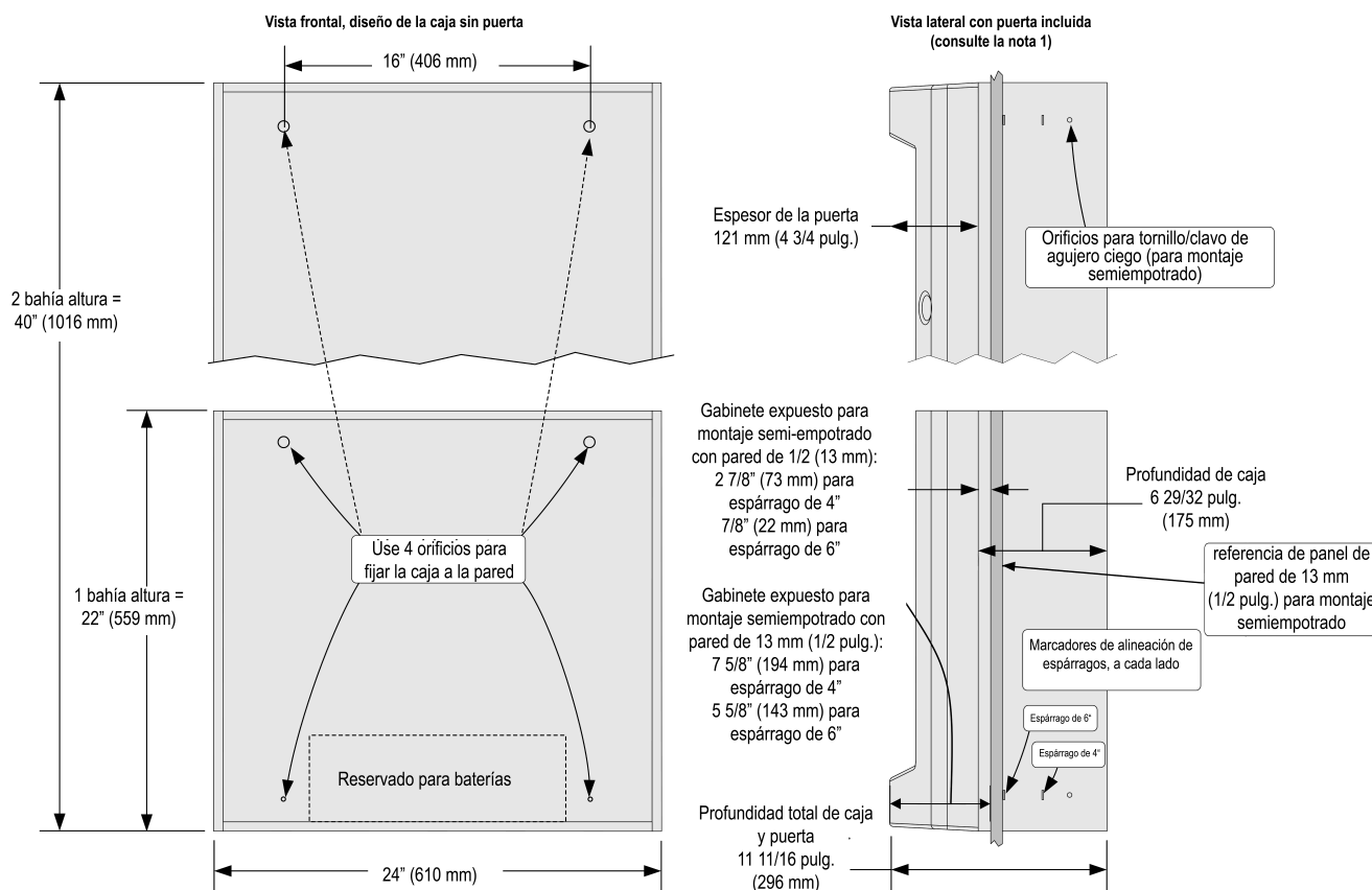
Figura 11: Referencia de medidas del gabinete
