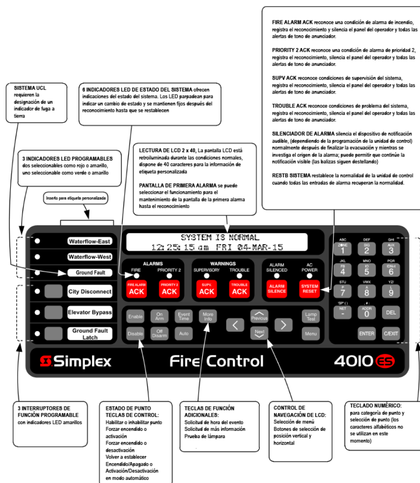
Figura 9: Características de la interfaz del operador
