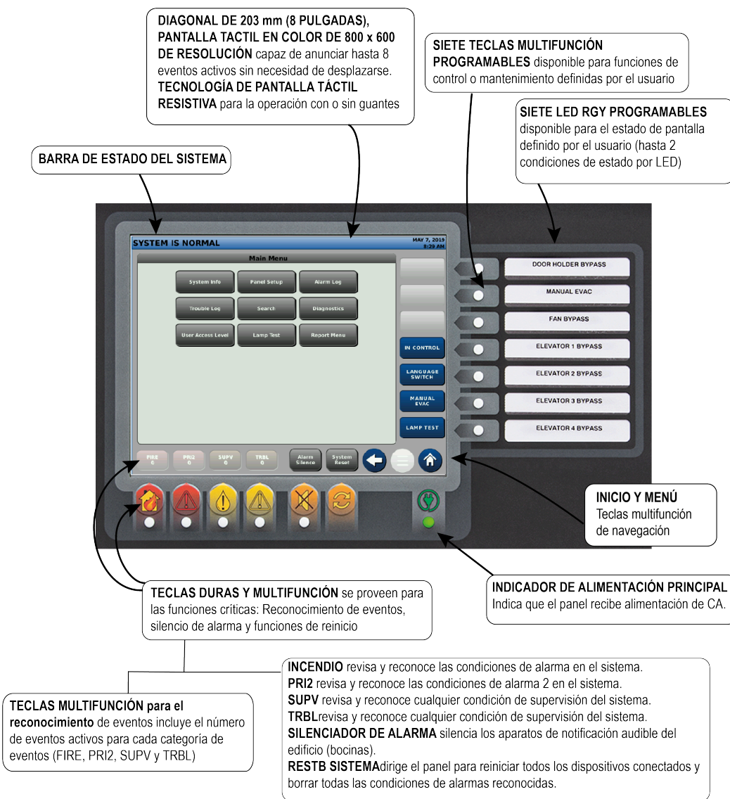
Figura 2: Interfaz de Operador de Pantalla Táctil ES
