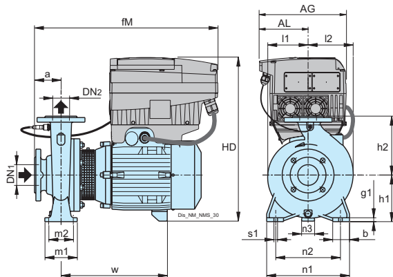
Bridas EN 1092-2
