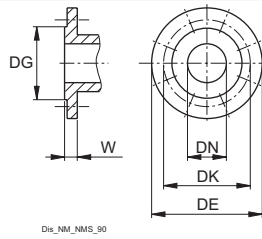
Bridas EN 1092-2
