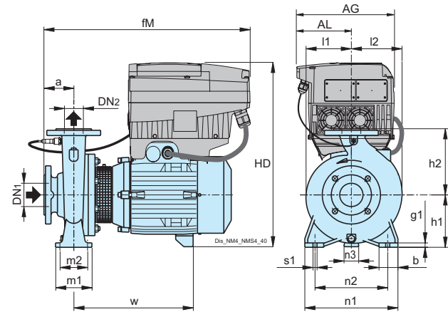
Bridas EN 1092-2
