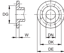
Bridas EN 1092-2
