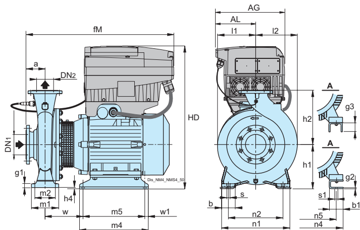
Bridas EN 1092-2
