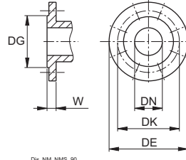
Bridas EN 1092-2
