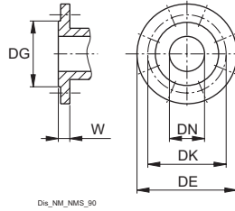
Bridas EN 1092-2
