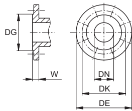
Bridas EN 1092-2
