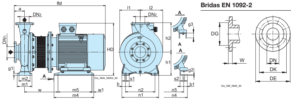
Bridas EN 1092-2
