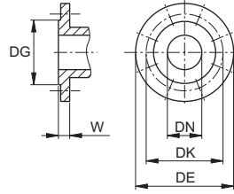
Bridas EN 1092-2
